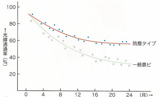
光線透過率の比較（直進光）
